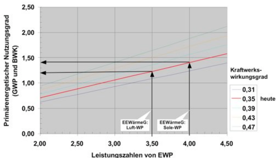
Abb. 1-6 Umrechnungsdiagramm für Leistungszahlen (Elektro-WP) und primärenergetischem Nutzungsgrad als Funktion des Kraftwerkswirkungsgrades (inkl. Netzverluste)
